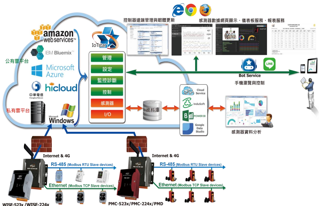
圖 1-1：IoTstar 系統架構圖
