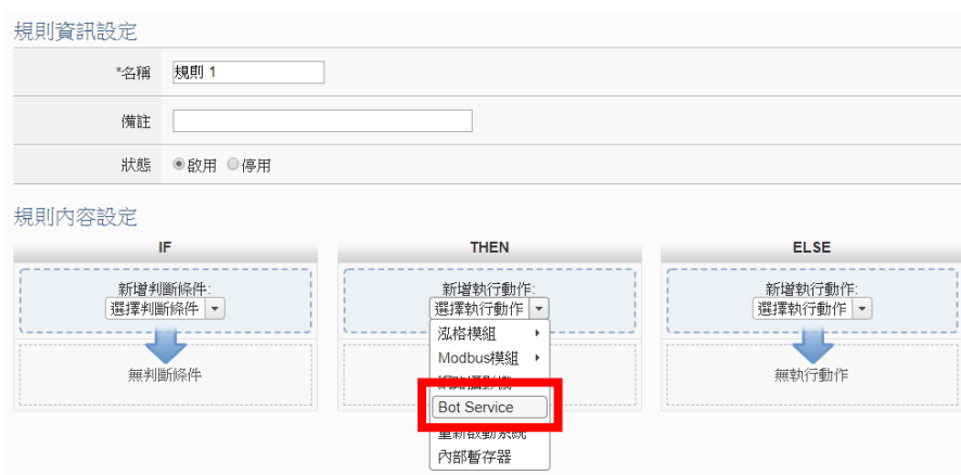
圖 2-32：WISE 網頁－Bot Service 訊息規則設定
