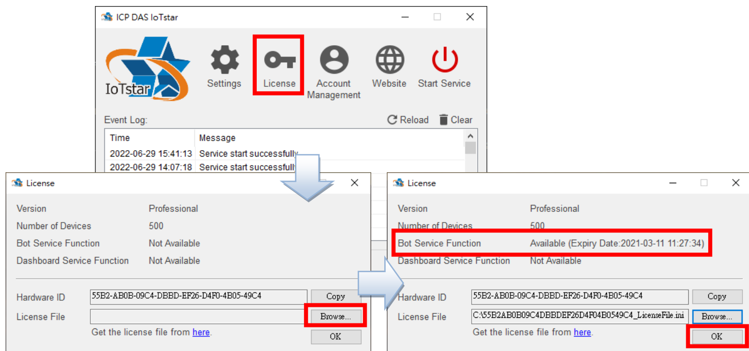
圖 2-13：取得並啟用試用服務的 License File (4)
