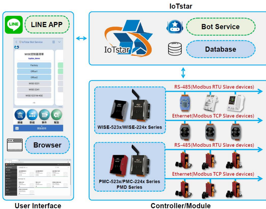
圖 1-2 : IoTstar Bot Service 架構圖
