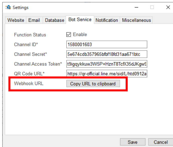
圖 2-20 : IoTstar 軟體 Bot Service 功能設定及啟動 (3)
