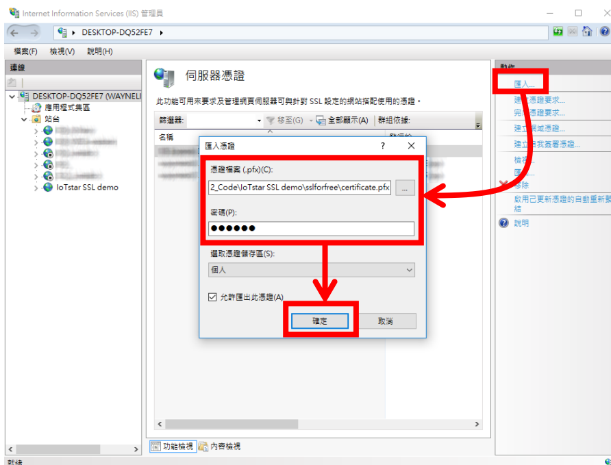
圖 2-25：於 IIS 匯入 SSL 憑證
