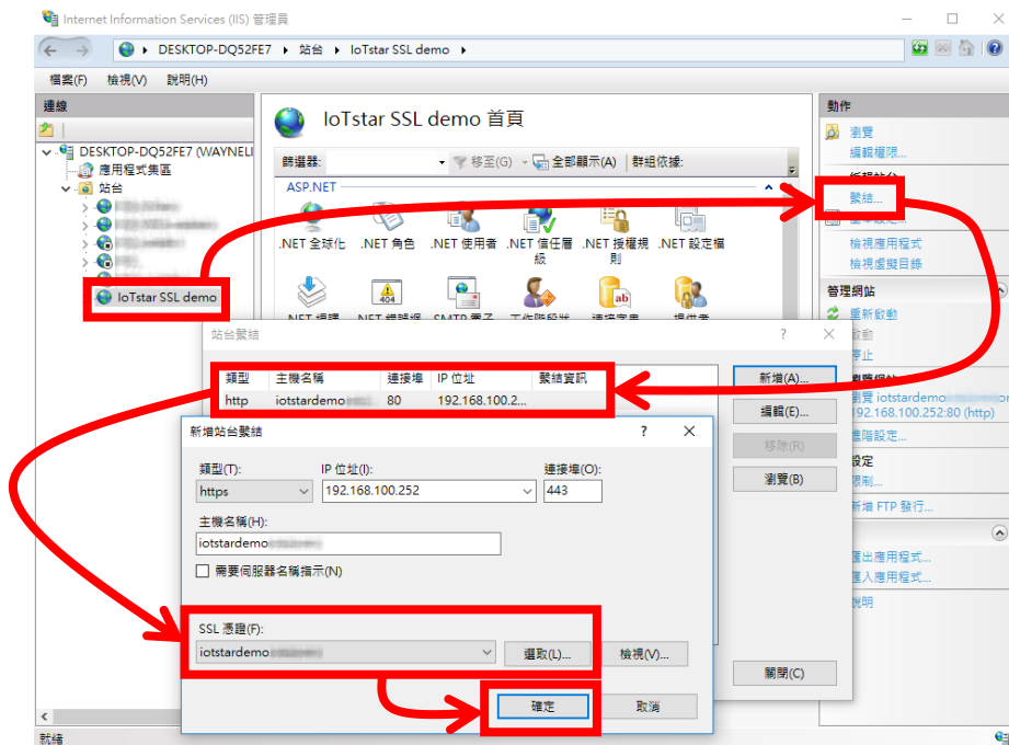
圖 2-26：於 IIS 上啟用 IoTstar 網站的 HTTPS 連線
